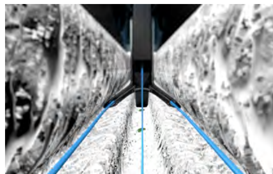
Figure 2. FurrowJet Placement
